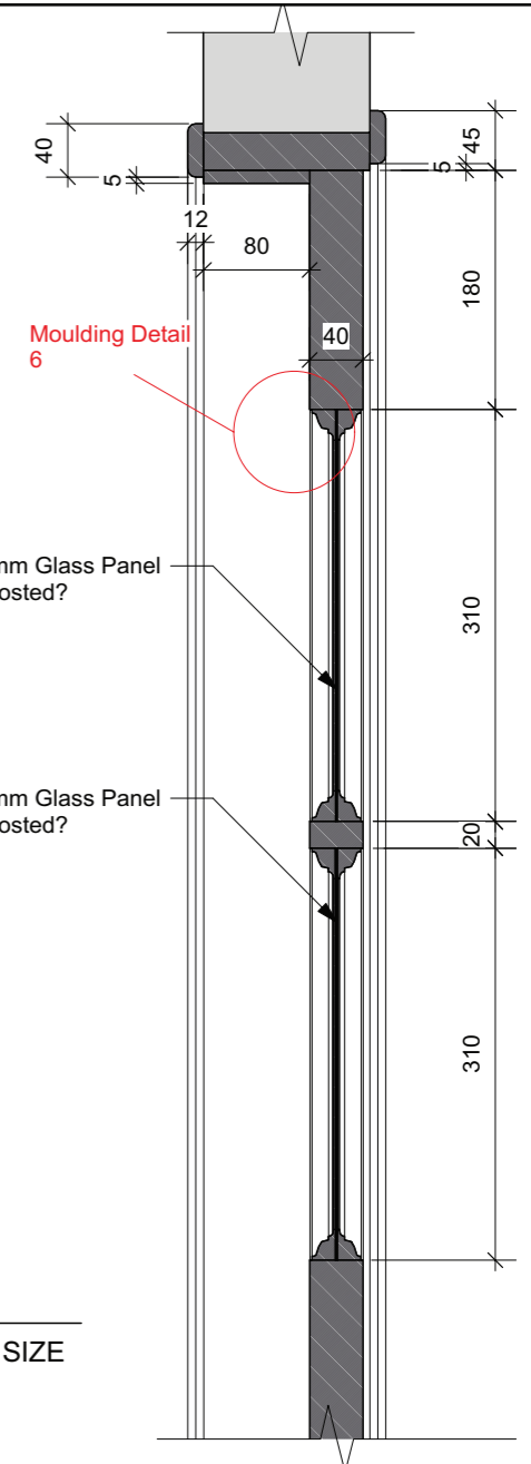
5 Section Detail Scale: 1:5
