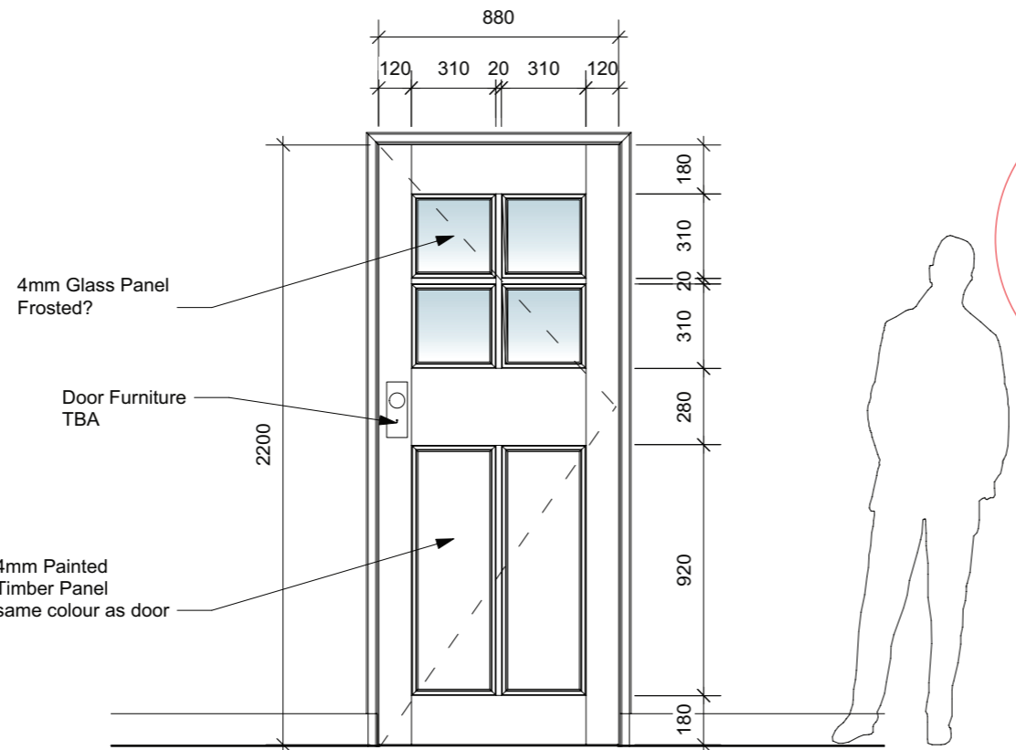
2 Front Elevation Scale: 1:20
